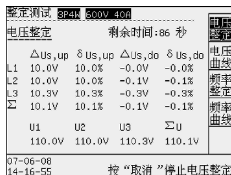
图 9-1 整定测试
