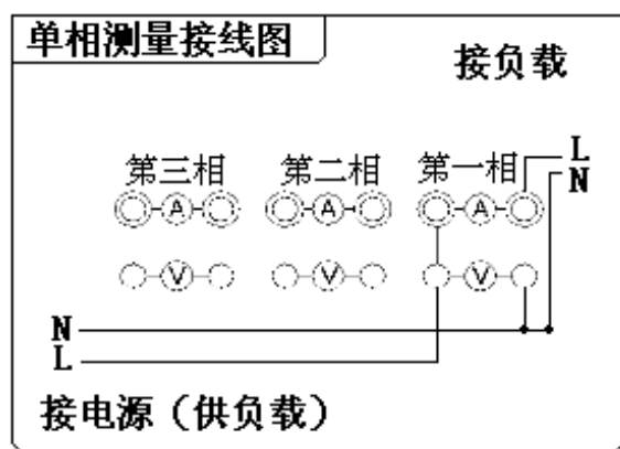
图 4-4 单相接线图
