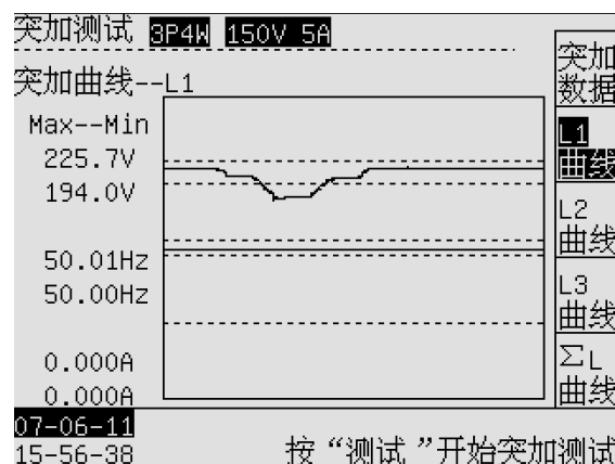
图 11-2 突加测试-L1 曲线
