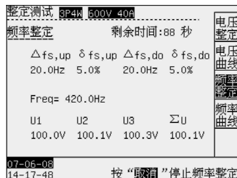
图 9-3 频率测试
