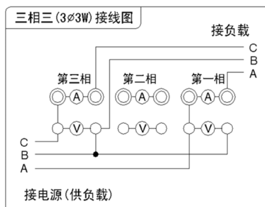
图 4-5 3P3W 接线图
