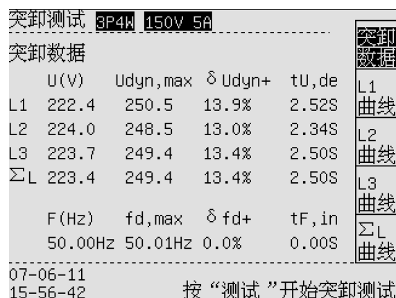
图 12-1 突卸测试数据
