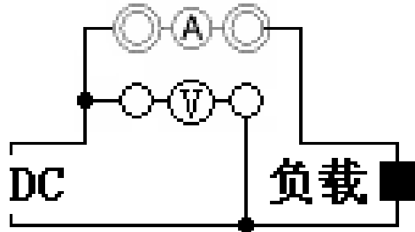
图 4-12 直流信号接线图
