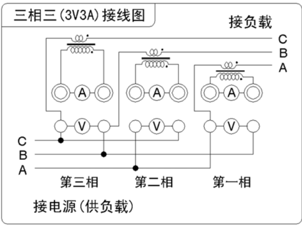
图 4-11 三相三线（3V3A—CT）接线图
