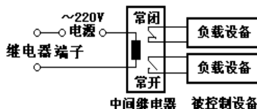
图 4-3 继电器端子的扩展使用
