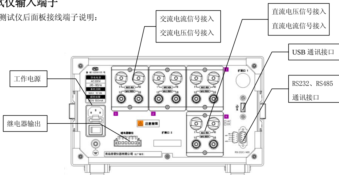
图 4-1 测试仪后面板
