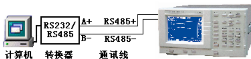
图 15-1 测试仪与计算机通讯—RS485
