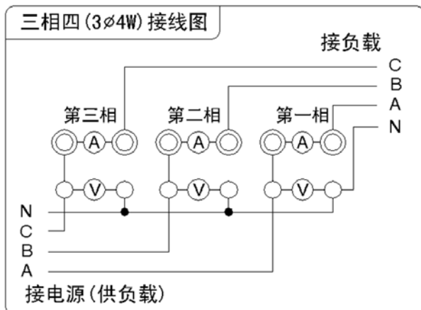
图 4-6 3P4W 接线图
