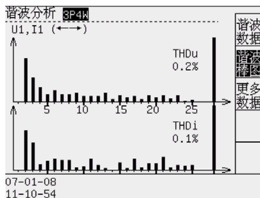
图 7-2 谐波棒图
