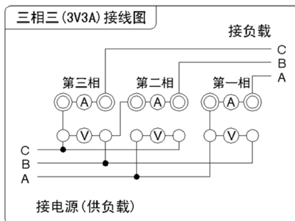
图 4-7 3V3A 接线图
