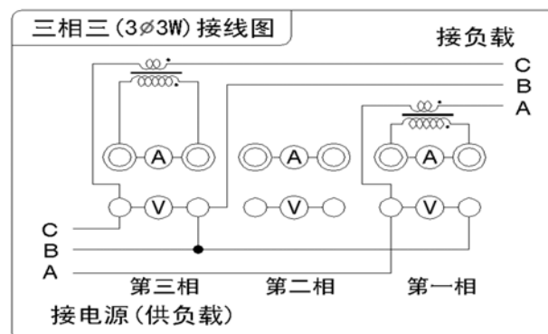
图 4-9 三相三线 (3P3W--CT) 接线图
