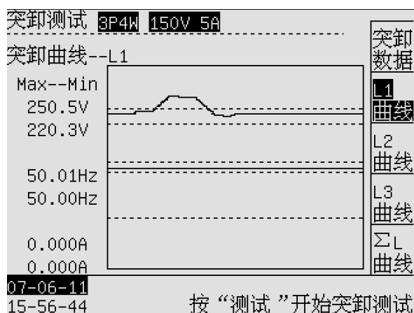
图 12-2 突卸测试-L1 曲线
