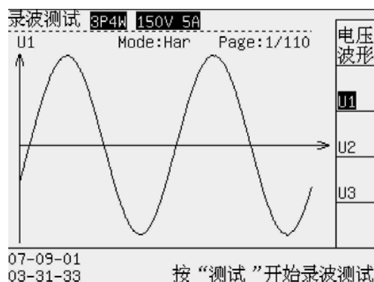
图 13-2 U1 录波曲线
