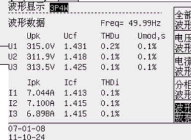
图 6-5 波形数据
